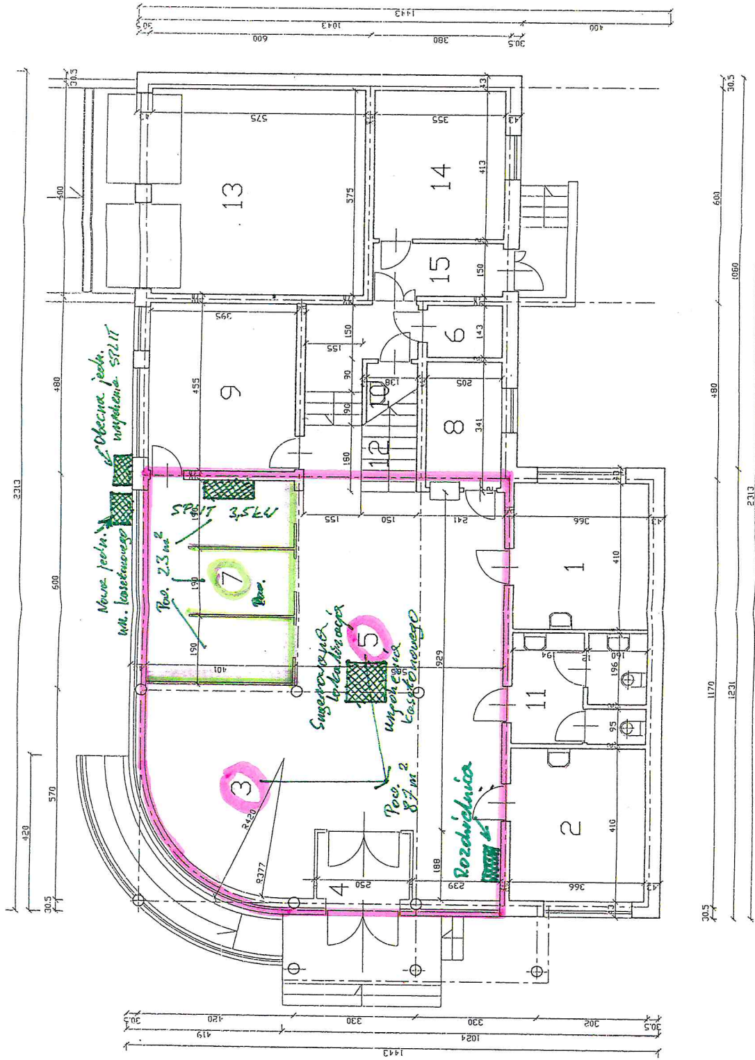
RZUT PARTERU-PIWNIC 1:100
