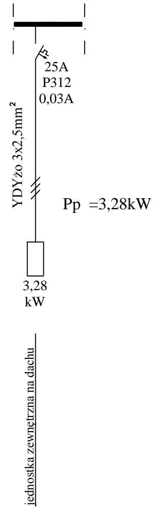
T4 - Fragment rozdzielnic obwody projektowane
