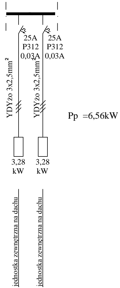
RG - Fragment rozdzielnic obwody projektowane
