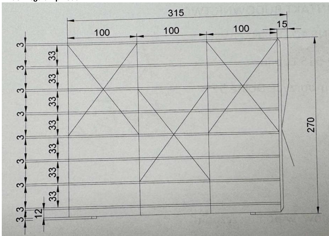
Widok regału z przodu
